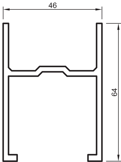
No : 5182 Kompozit Panel Prf. 1,230 kg/m
