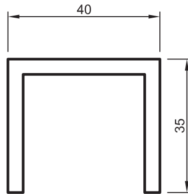
No : 839 U Profili 1,110 kg/m
